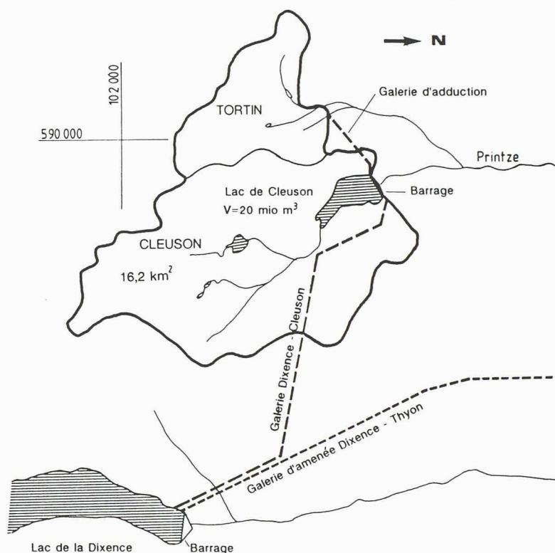
Fig. 1. – Barrage de Cleuson: situation d'ensemble de l'aménagement
