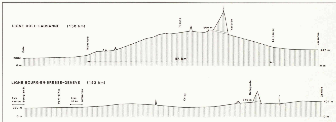
Projets de lignes à grande vitesse transjures: profils en long.
