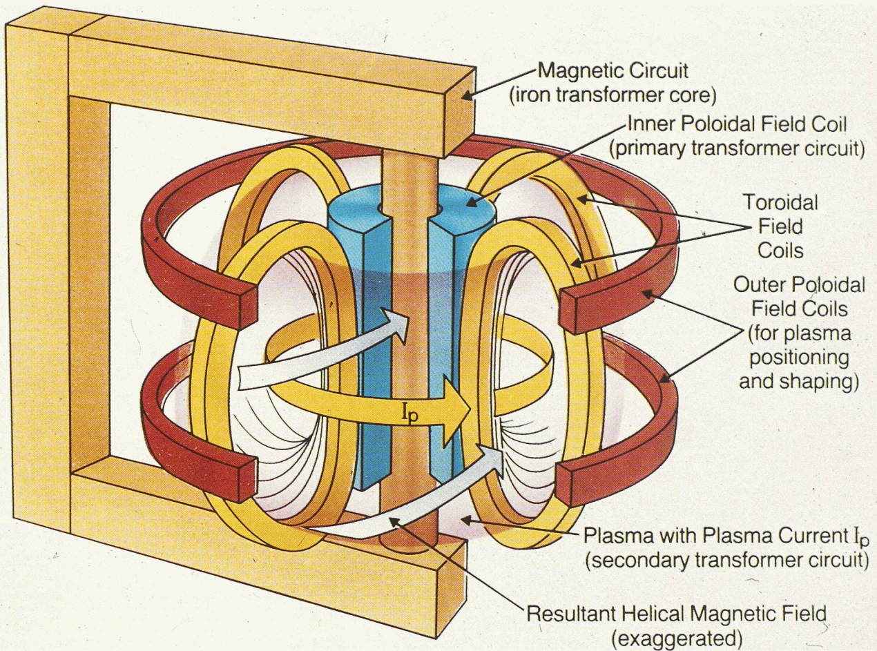
Fig. A. - Schéma de fonctionnement du tokamak.
