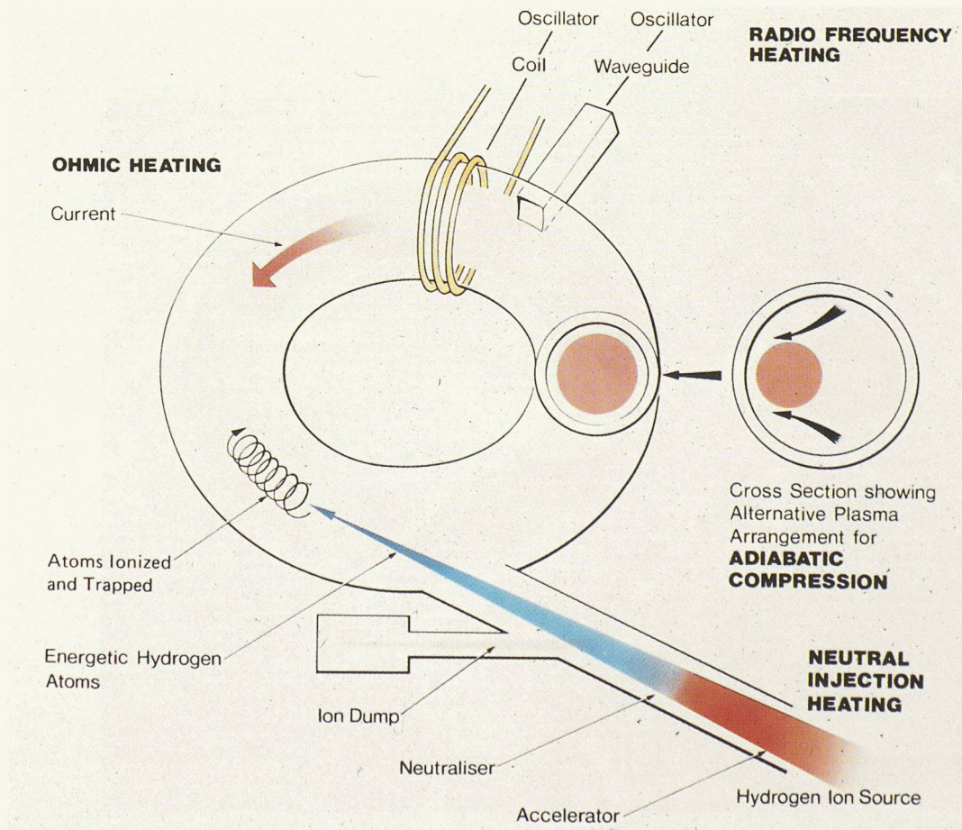
Fig. B. - Représentation schématique des méthodes de chauffage du plasma.
