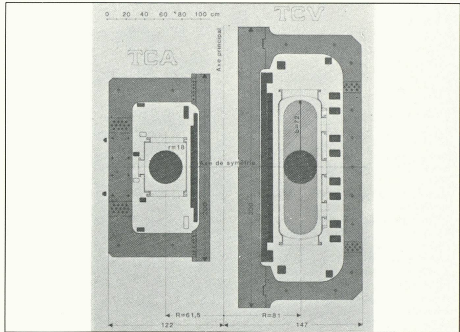
Fig. 7. – Comparaison du TCV (tokamak à configuration variable) avec le TCA. Caractéristique principale du nouveau projet TCV: sa capacité à changer la forme et les dimensions de la section du plasma.
