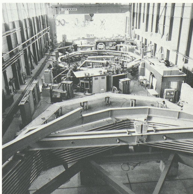
Aménagement de l'un des deux ateliers de bobinage, équipé pour la manutention de pièces de 60 t.
