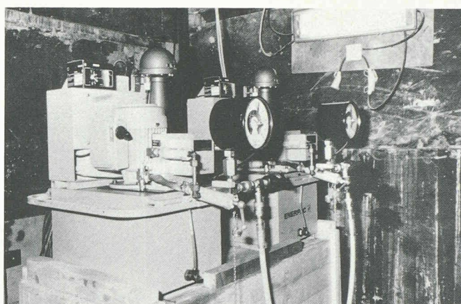
Fig. 7. — Les pompes hydrauliques Enerpac BPE-30343 utilisées pour alimenter l'ensemble des 148 vérins supports. On aperçoit clairement leurs manomètres, minuterics et alarmes acoustiques.
