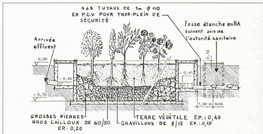
Fig. 3. — Coupe d'un plateau absorbant. Le trop-plein éventuel est évacué dans un réseau d'épandage en sous-sol. Tiré de Pratiques de l'assainissement des agglomérations, H. Guerrée, Ed. Eyrolles.
