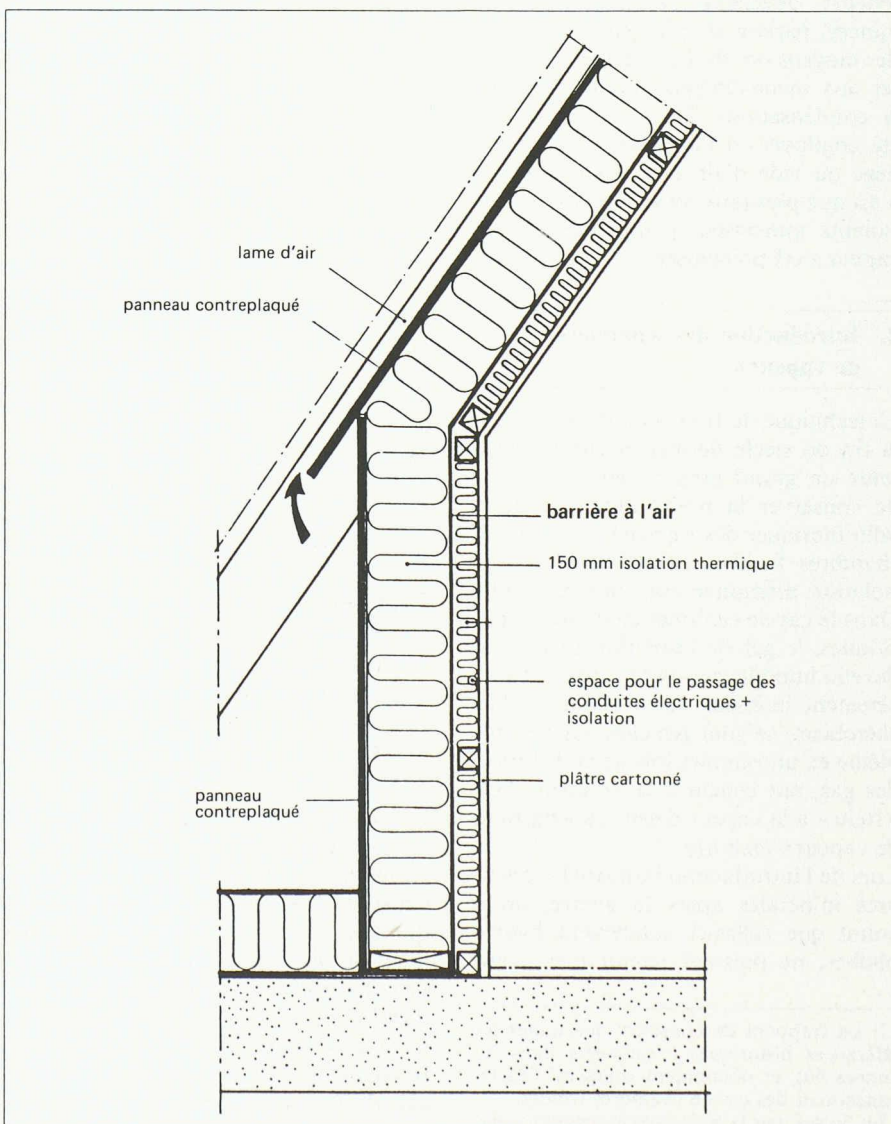
Coupe d'une façade. Extrait de Airtightness and thermal insulation, éditions Bygghälseskraden, Stockholm, 1980.
