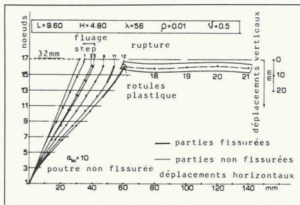
Fig. 14. Déplacements de la colonne de gauche et de la poutre dans la deuxième histoire de charge (avec fluage et imperfection initiale)
