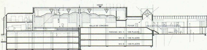
Maison de congrès, coupe
