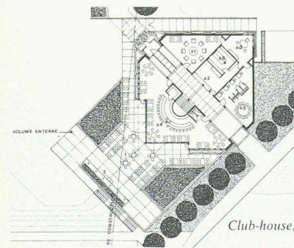
Rez-de-chaussée supérieur 1: 1000
