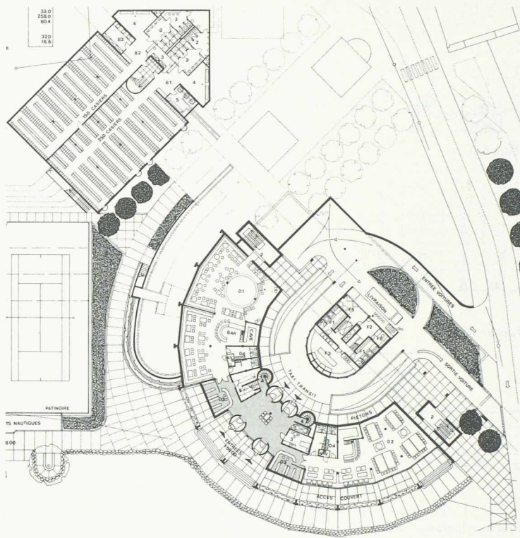
Rez-de-chaussée inférieur 1: 1000
