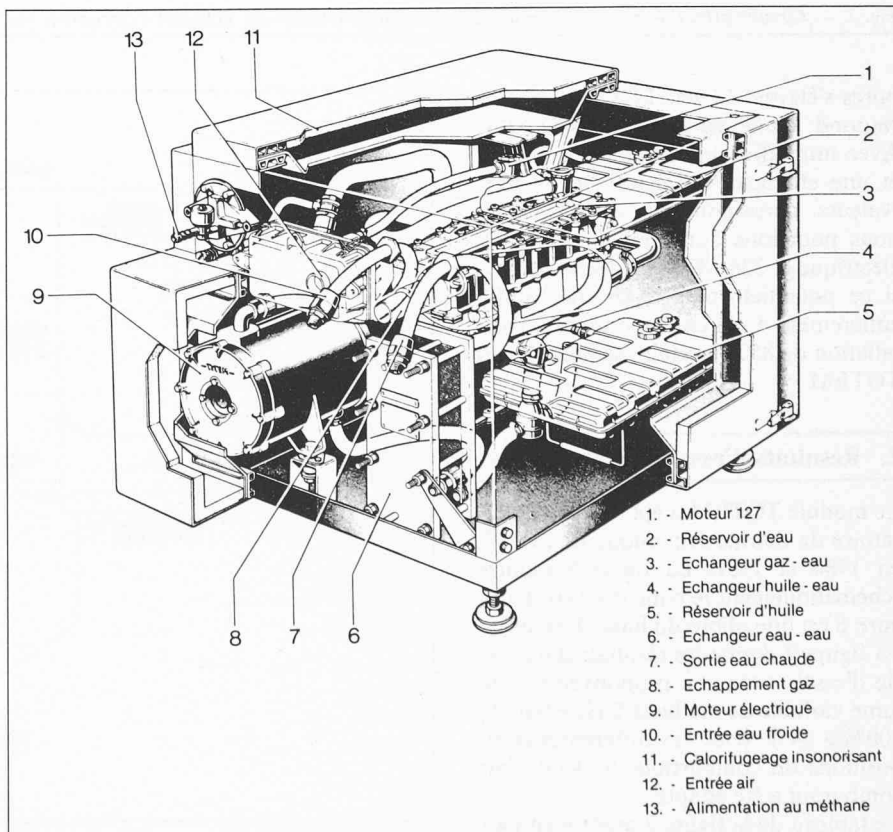
Fig. 2. — Eclaté du TOTEM montrant ses différents éléments. (Document Fiat)
