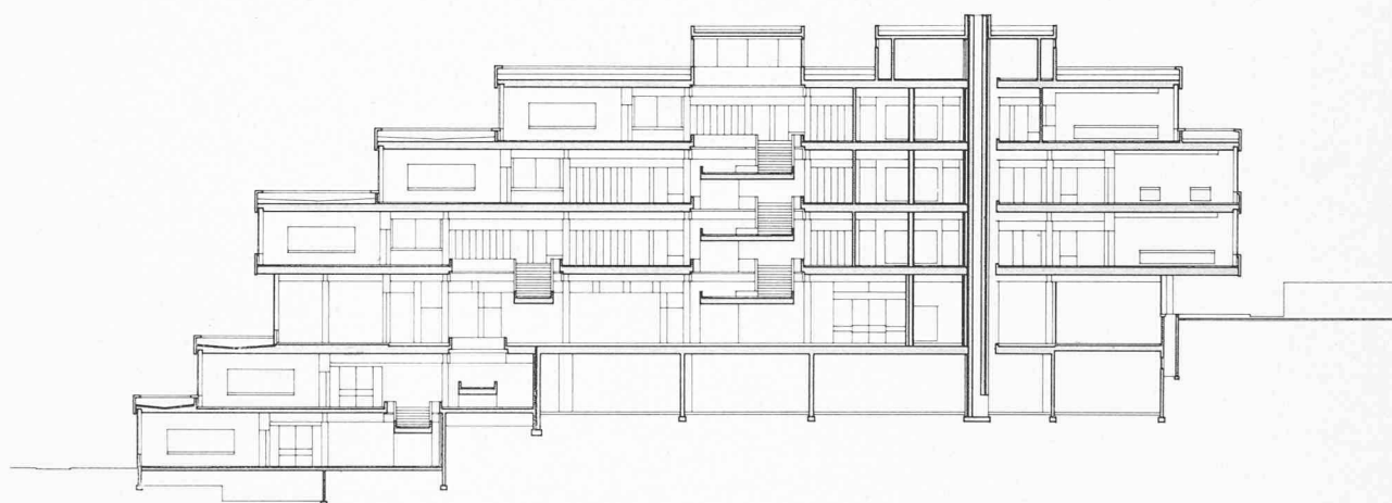
Fig. 11. — Coupe du bâtiment principal.
