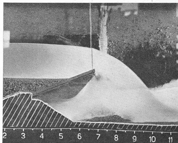
Fig. 21. — Débit total de la rivière : 150 \text{ m}^3/\text{sec} . Pression de purge : 4,5 \text{ m} (correspondant au niveau de retenue).
