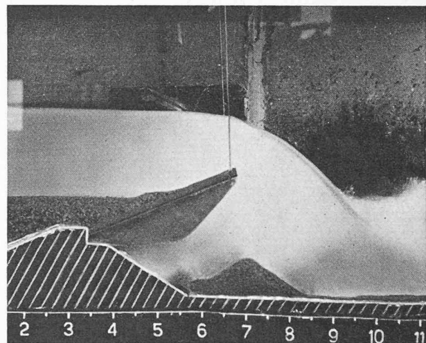
Fig. 22. — Débit total de la rivière : 150 \text{ m}^3/\text{sec} . Pression de purge : 10 \text{ m} .
