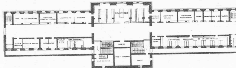
1 er sous-sol.
