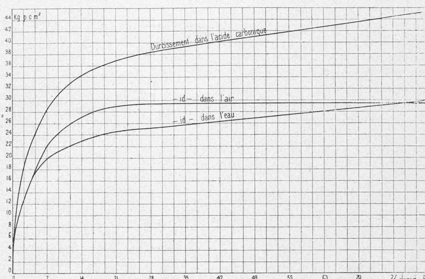
Fig. 4. — Influence du milieu sur le durcissement du ciment artificiel. Essais du laboratoire fédéral de Zurich.
