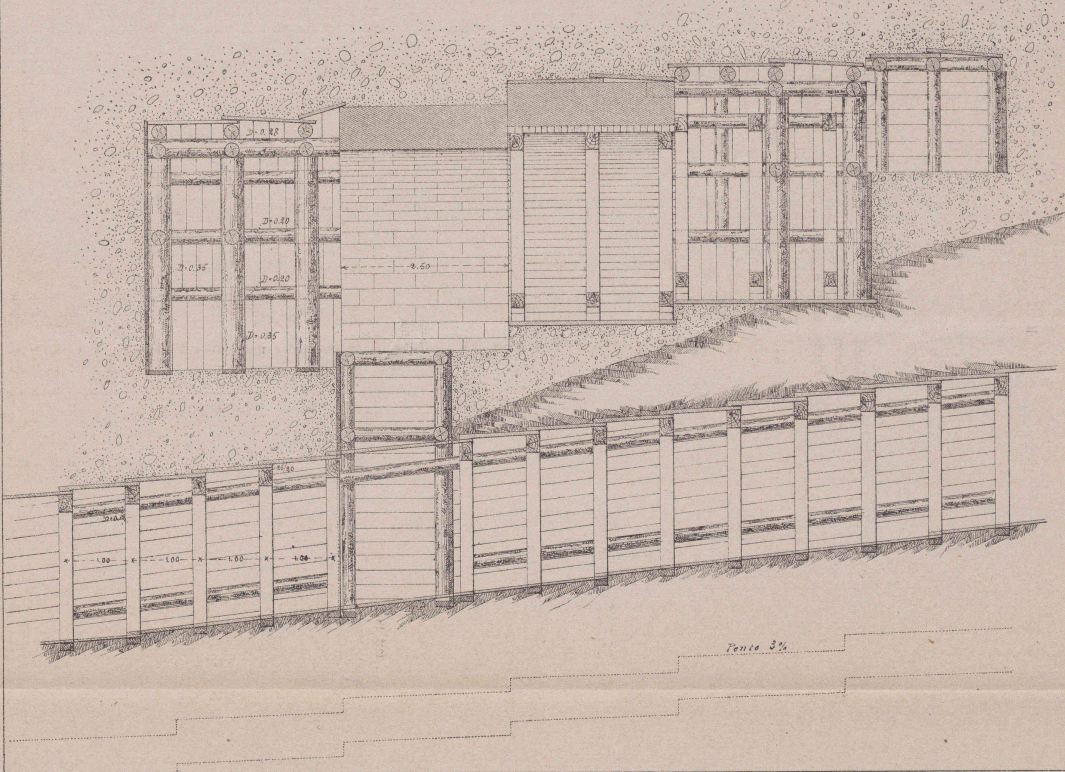
COUPE LONGITUDINALE
