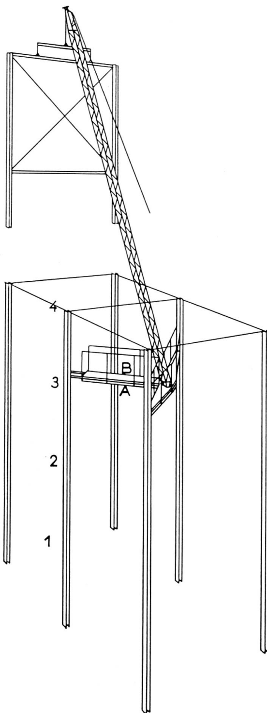
Fig. 3. Mât de montage haubané et mis en service.
