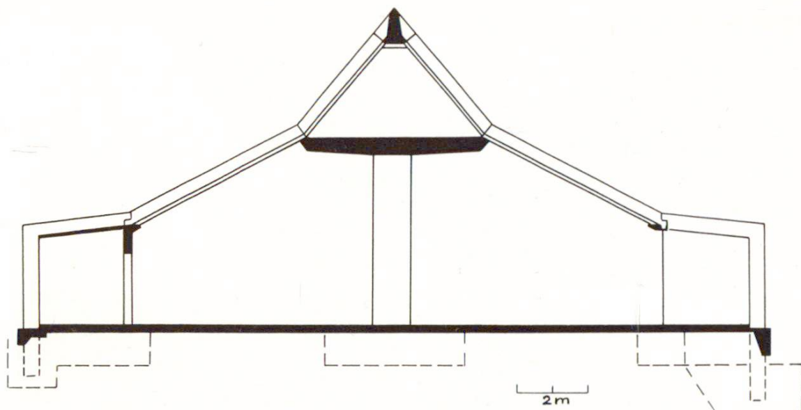
Fig. 5 Coupe schématique du pavillon.
