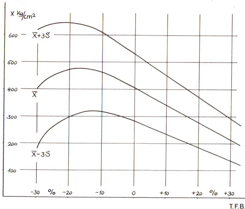
Fig. 2 Variations de la résistance moyenne à la compression du béton dues à des erreurs de mesure de la quantité d'eau ( \pm \% \text{ eau} ). Domaine de variation limité par le triple de l'erreur quadratique moyenne ( \pm 3 S ) ; le 99,7 % de tous les résultats se trouvent dans ce domaine selon Vironnaud (Bibl. 1)
