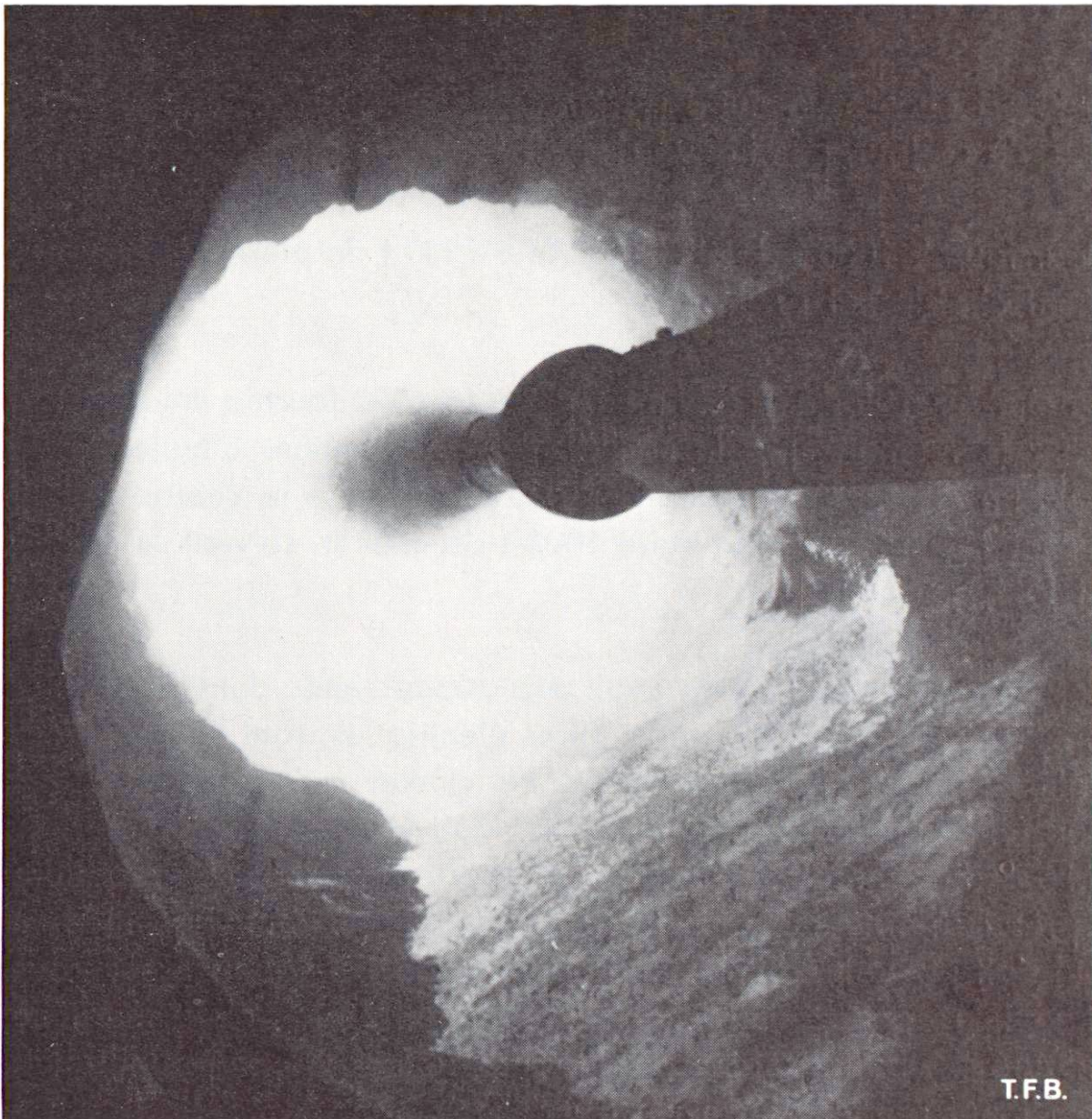
Fig. 3 Vue à l'intérieur d'un four rotatif, par sa partie inférieure, avec la tuyère d'alimentation en poussier de charbon. Le clinker, en couche inclinée sous l'effet de la rotation du four, roule lentement vers la sortie
