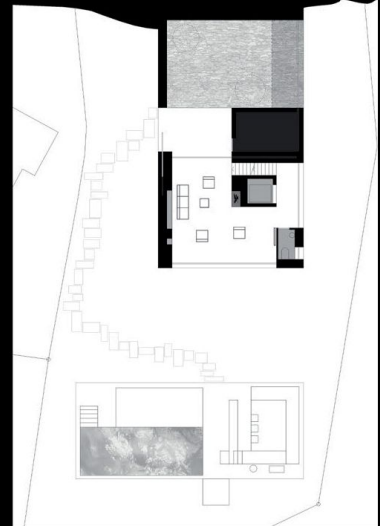
Pianta livello 3
