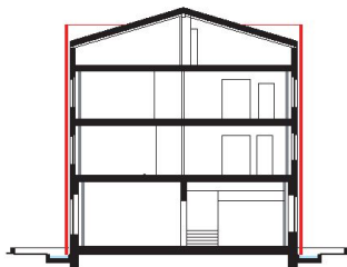
Sezione trasversale
