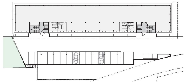
Pianta terzo piano
