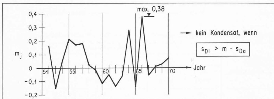
Bild 8. Verhältnis m_j = A_j/B_j für die Jahre 1950–1970 für das Klima Zürich ( \phi_i = 50\% )
