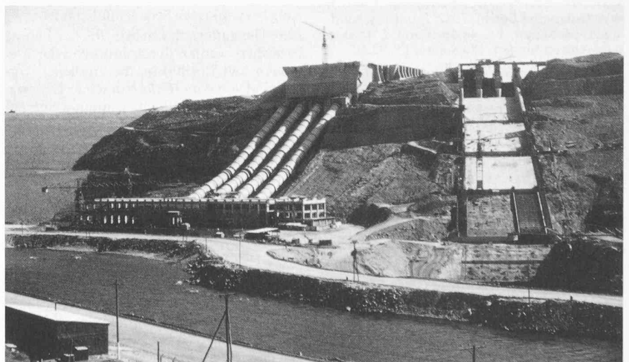
Wasserkraftanlage Alicura, Argentinien. Im Hintergrund links der nahezu vollendete Schüttdamm, in Bildmitte Druckleitungen und Zentrale ( 4 \times 250 = 1000 MW) und am rechten Bildrand Hochwasserentlastung
