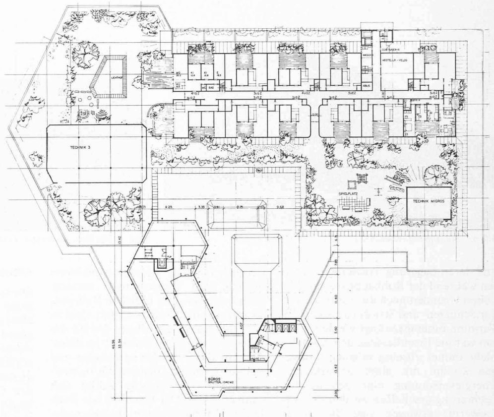
Bild 5. Grundriss Dachaufsicht
