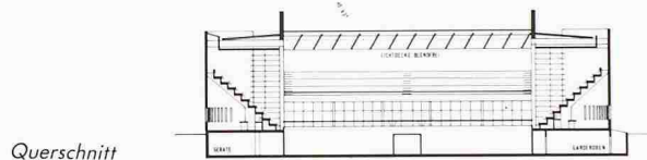
Querschnitt
