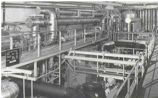
ETH-Wärmepumpenanlage Walche
