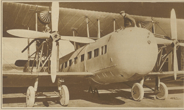
Die Maschine auf dem Gebiete der Flugtechnik darft das diese Tage in England fertiggestellte Flugzeug mit Rotationsmotor als Vorbild. Der Apparat hat eine Tragkraft von 22 Personen und seine Motoren zusammen nicht weniger als 12000 Pferdekräfte.
