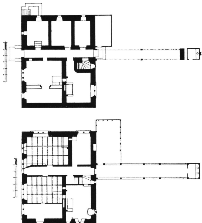
Abb.10 Schmittens, Herrenhaus de Weck in Bluemisberg aus den 1620er Jahren. Grundrisse des Erd- und Obergeschosses mit Querkorridor und Latringalerie.
