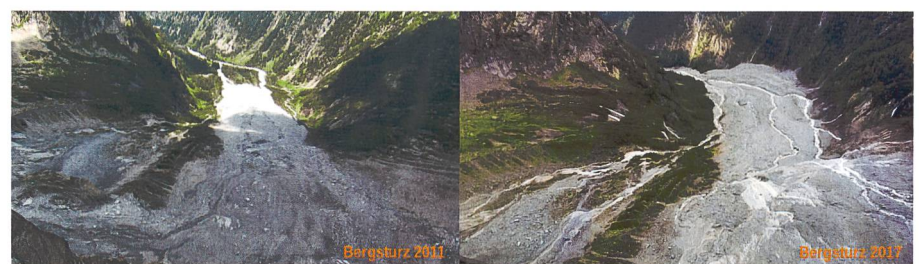
Bild 2. Ablagerungen der Bergsturzereignisse am Piz Cengalo von Dezember 2011 (links) und August 2017 (rechts) im Vergleich.
