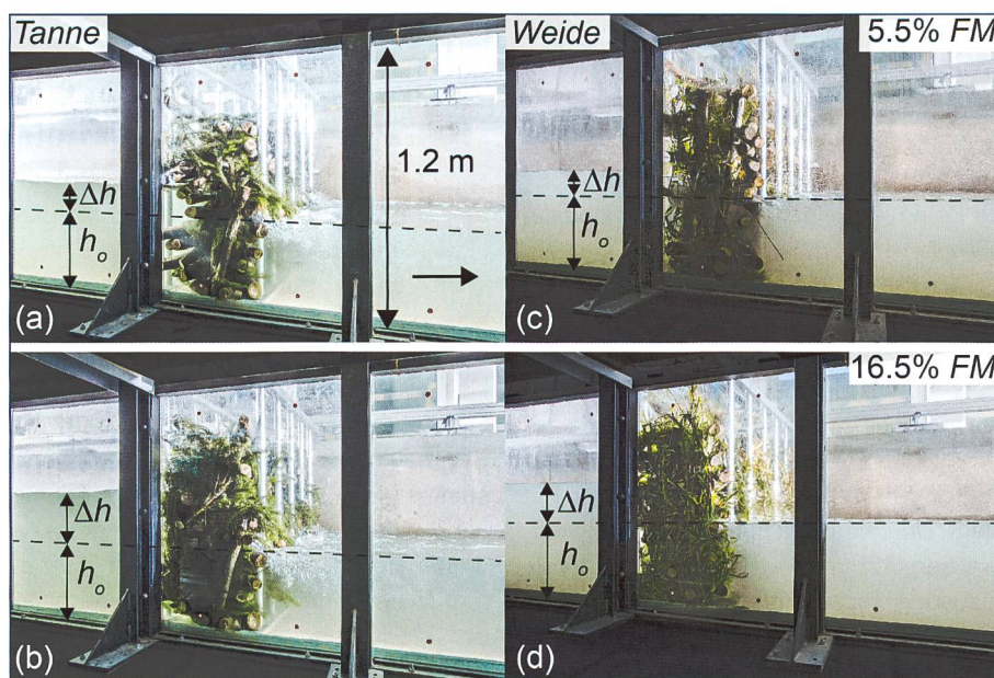
Bild 6. Aufstau \Delta h infolge Schwemmholtzverklauung mit zunehmendem FM -Anteil ( F_o = 0.3 , h_o = 0.36 \text{ m} , a = 4.2 , L_A = 0.50 \text{ m} , und d_L = 65 \text{ mm} ); (a–b) Tannenzweige und (c–d) Weidenäste.
