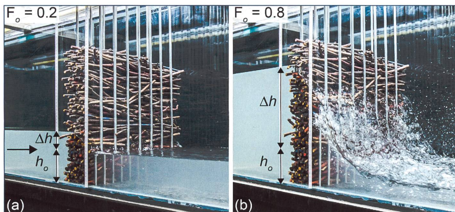
Bild 4. Aufstau \Delta h infolge Schwemmholtzverklauung für (a) F_o = 0.20 versus (b) F_o = 0.80 ( h_o = 0.10 \text{ m} , a = 3.3 , L_A = 0.10 \text{ m} und d_L = 7 \text{ mm} ).
