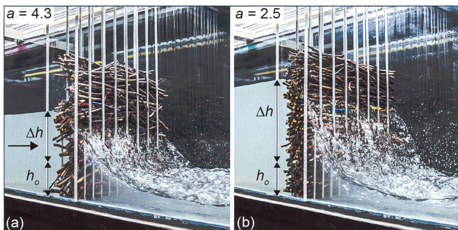
Bild 5. Aufstau \Delta h infolge Schwemmholtzverklauung für (a) a = 4.3 versus (b) a = 2.5 ( h_o = 0.10 \text{ m} , F_o = 0.8 , L_A = 0.10 \text{ m} und d_L = 7 \text{ mm} ).
