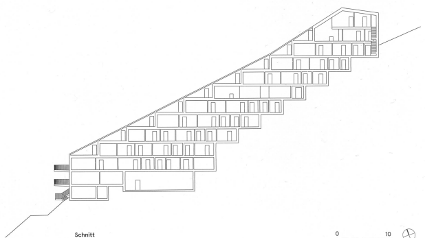
Schnitt
