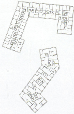
1.-4. Obergeschoss
