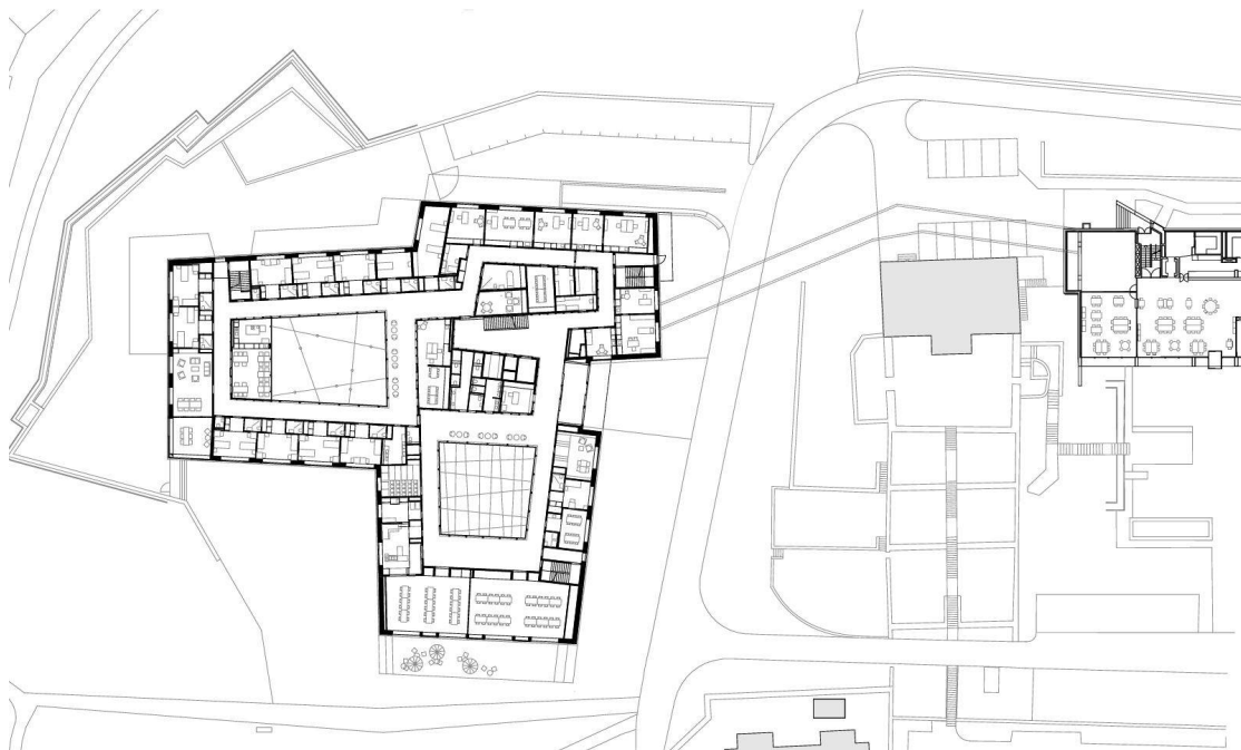
Erdgeschoss 0 5 10
