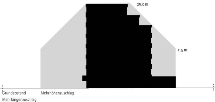
Figur des Wohnhauses mit Mantellinie
