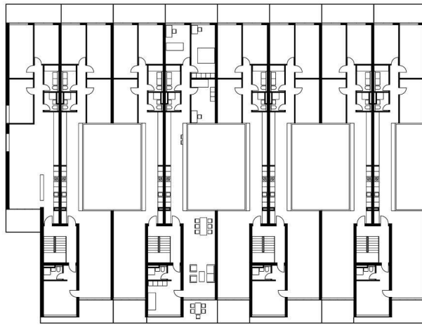
Obergeschoss (Wettbewerb)
