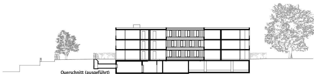
Querschnitt (ausgeführt)
