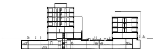
Querschnitt
