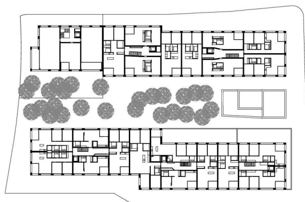
2. + 3. Obergeschoss
