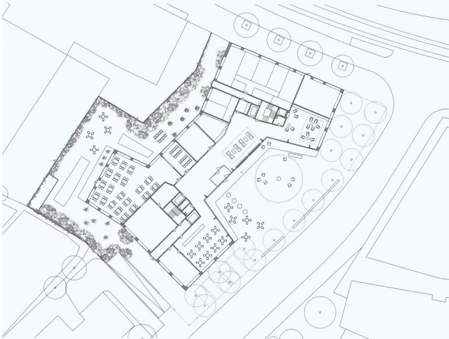
Grundriss EG
