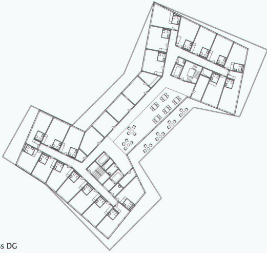
Grundriss DG
