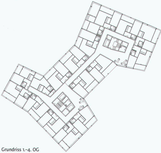
Grundriss 1.-4. OG
