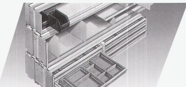
Austauschbares Lista-Schubladensystem
