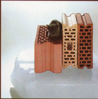
Wärmeisolierend
