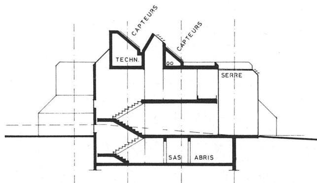
33 Coupe/Schnitt.
