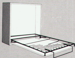
7. Bettlift für Doppelbett mit abklappbarem Kopfteil und Federbespannung.
