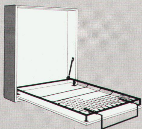
4. Bettlift für Doppelbett mit Federbespannung.
