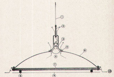
1 Kabel; 2 Regulierung der Höhe; 3 Lampe 100 W; 4 Regulierung der Lage; 5 Lüftung; 6 Plastikkuppel, rauchgrau; 7 Platte; 8 Gummifüße; 9 Auflageebene; 10 Lüftung
