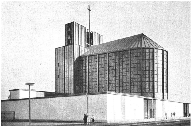
1928. Stahlkirche auf der Presseausstellung in Köln von Otto Bartning, Arch. BDA. 1930 abgebrochen, in Essen wieder aufgebaut; 1943 zerstört (Aus Hans K. F. Mayer: Der Baumeister Otto Bartning und die Wiederentdeckung des Raumes. Verlag Lambert Schneider, Heidelberg, 1951) Eglise en acier à Cologne | The steel church in Cologne, destroyed 1943
