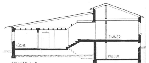
SCHNITT A-B
