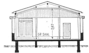
SCHNITT E-F
