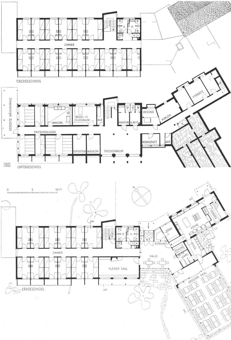
Grundrisse Hauptgebäude 1:400 | Plans du bâtiment principal | Plans of the main building
