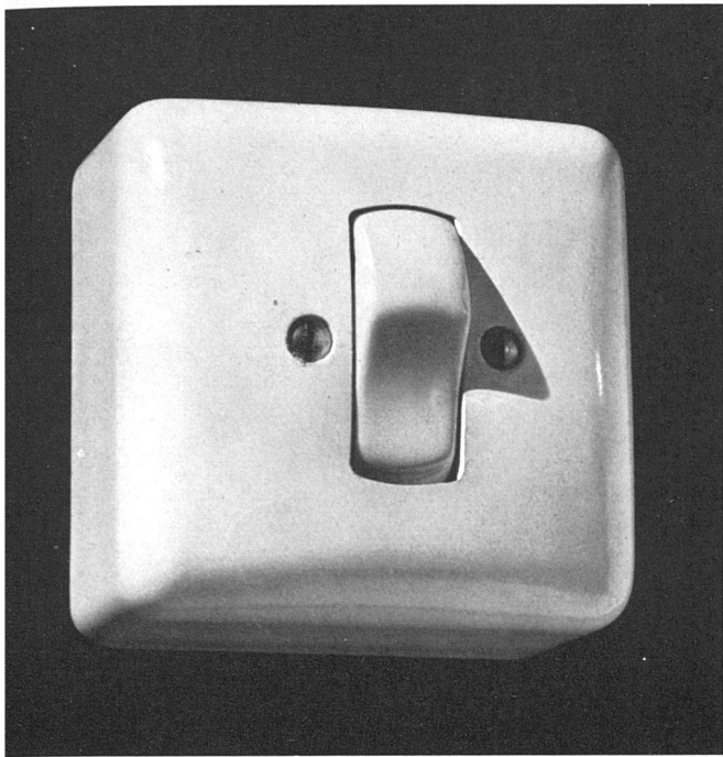
Leppbalkenschalter 1:1, viereckig für Zusammenbau / Interrupteur à scule pour montage en bloc / Square lever switch for block assembly
