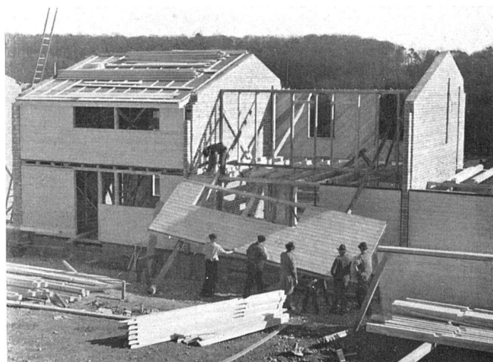
Vorfabrizierte Fassadeneinheiten zwischen Backsteinmauern (Siedlung Bocksrüt, 1942/43, Architekt BSA W. Vetter, Lausanne) / Eléments façade préfabriqués, entre murs de briques / Prefabricated façade unit between brick cross walls
