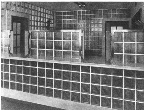
Schalteranlage in der Uhrenfabrik «Eterna», ausgeführt mit Glasbausteinen Verliith/Vitrablock Nr. 120, 20/20/5 cm
