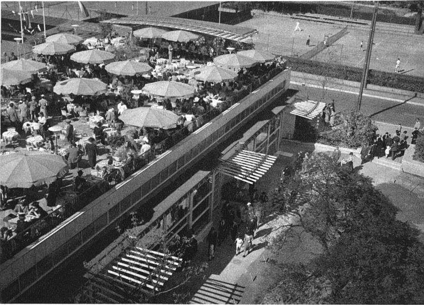
Kongresshaus Zürich. Terrassenrestaurant über dem Gartensaal, am östlichen Kopfe gegen die Clariden-Strasse gedeckte Estrade für das Orchester, gegen den Garten die Lattenvordächer der Eingänge zum Gartensaal, aufgehängt an zarten Gitterträgern (die auf S. 359 sichtbare Bambusrohrung fehlt noch). Die Dachterrasse fasst rund 700 Sitzplätze, der Garten gegen den Alpenquai 500.
