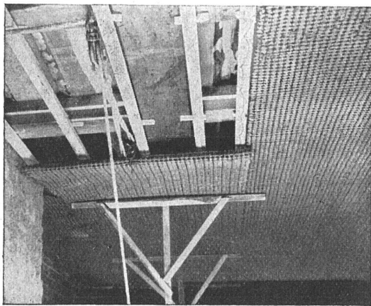
Rissfreie Drahtziegeldecken
