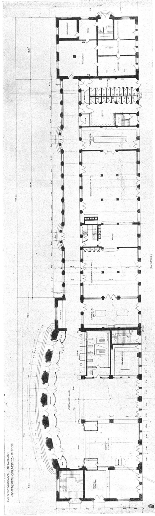
Bahnhof St. Gallen, Fassade nach der Geleiseseite und Parterregrundriss
